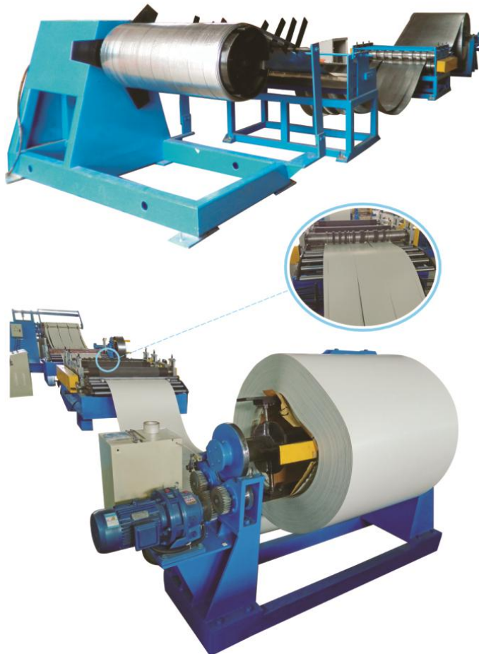
0.2-2.0毫米薄板纵剪线 0.2MM-2.0MM THICK SIMPLE SLITTING LINE
